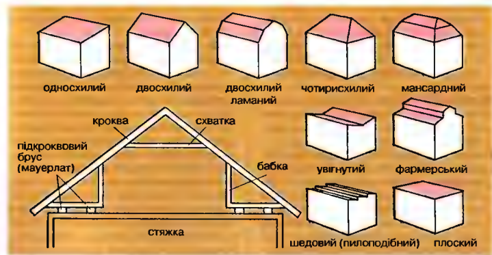
Покрівля Елементи покрівлі і види покрівель
